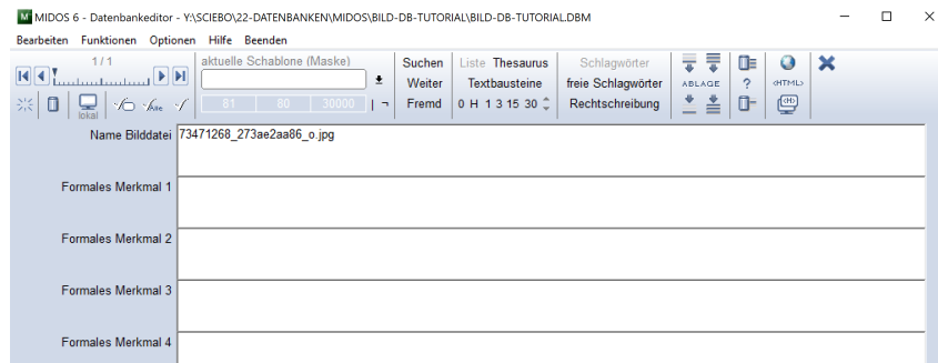
Abbildung 2: Midos 6 – Datenbankeditor
